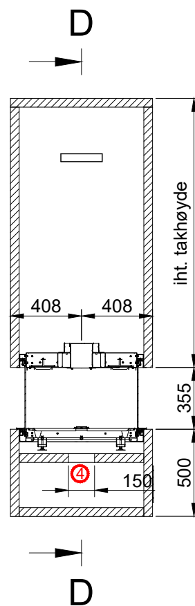
D-D (1:30)
