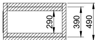
B-B (1:30)
